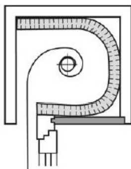
Einseitige Montage
